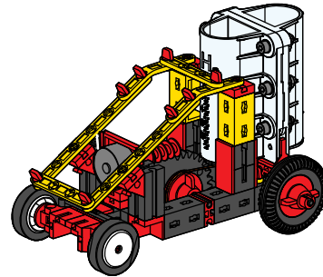
Brennstoffzellenfahrzeug / Fuel-cell vehicle / Véhicule à cellule électrochimique / Voertuig met brandstofcellen / Vehículo de células de combustible / Veículo de célula a combustível / Veículo a célula de carburante / Электромобиль с топливным элементом и солнечная станция / 燃料电池车 . . . . . 45
